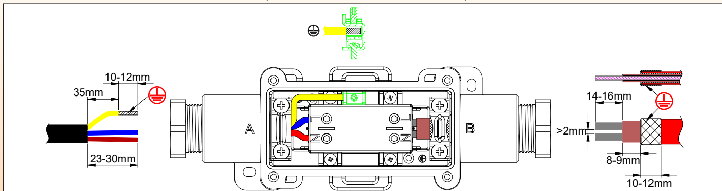
带一根电源电缆和一根发热电缆的型号
