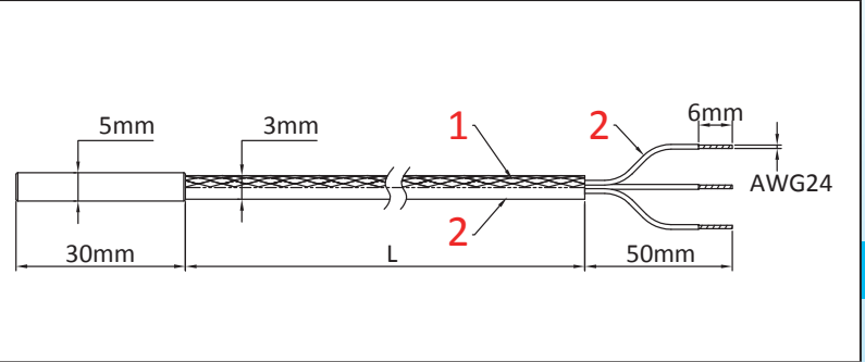
1: 红铜编织；2: 氟化乙丙烯
