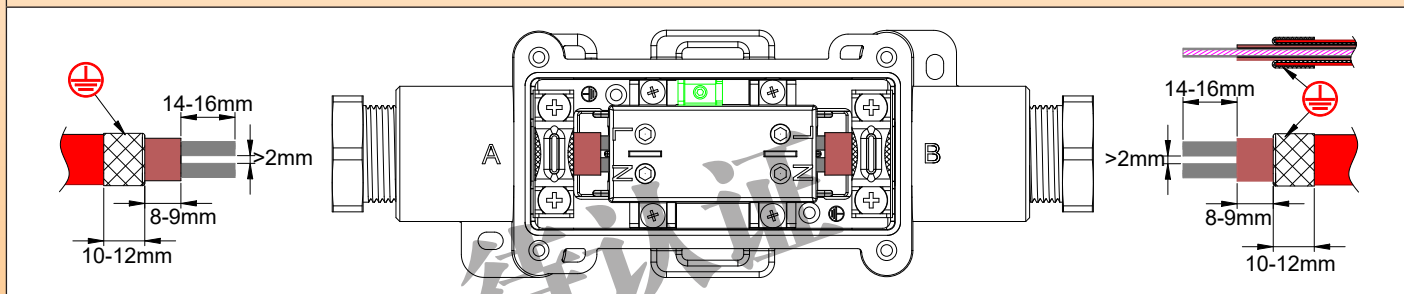
带两根发热电缆的型号
